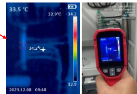
ตรวจสอบความร้อนสายกราวด์ MCCB 34.2 °C
