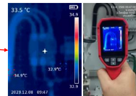
ตรวจสอบความร้อนสายเฟส MCCB 34.9 °C
