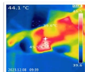
อุณหภูมิสายดิน INVERTER 45.5 °C 18SNPB-WIV01
