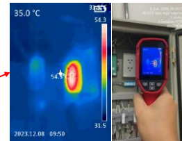
RTU FAN 54.3 °C
