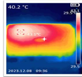
อุณหภูมิ Inverter NO.5 43.1 °C 18SNPB-WIV01
