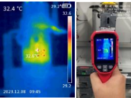
ตรวจสอบความร้อนสาย MCCB 32.6 °C
