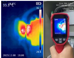
ตัวแปลงสัญญาณ 36.1 °C
